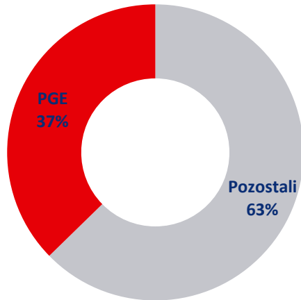
Udział PGE w mocach zainstalowanych w Polsce
